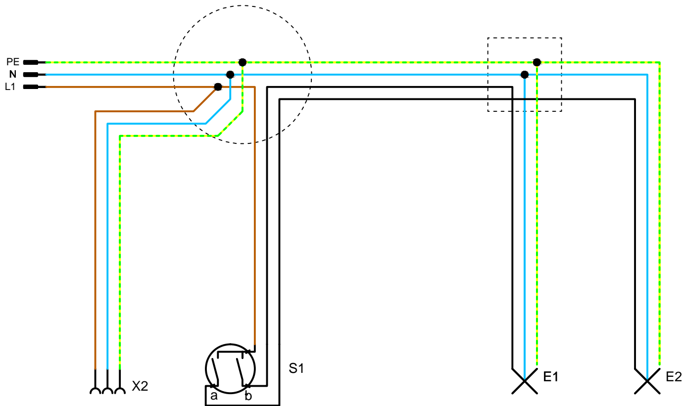
Bedradingschema
