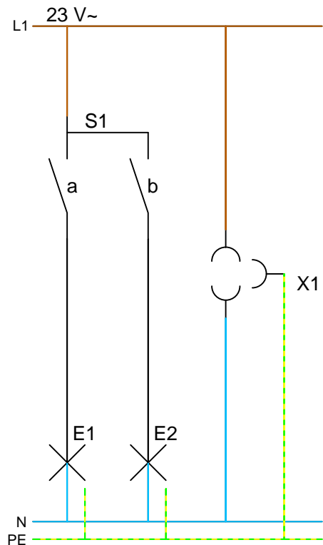
Stroomkringschema
